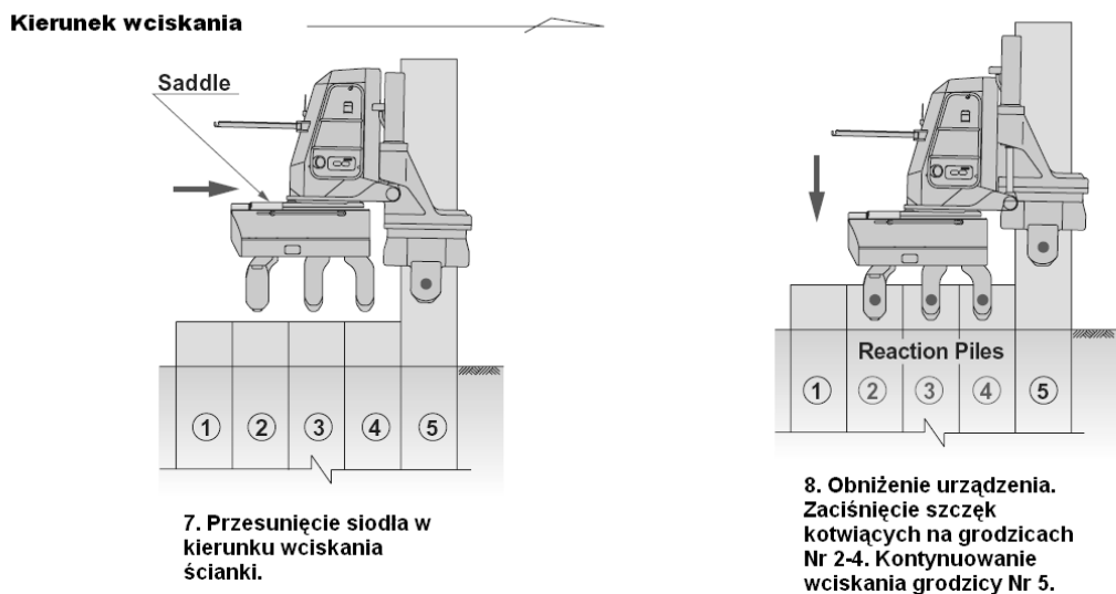
Rysunek 2. Procedura wciskania grodzic urządzeniem samokroczącym
